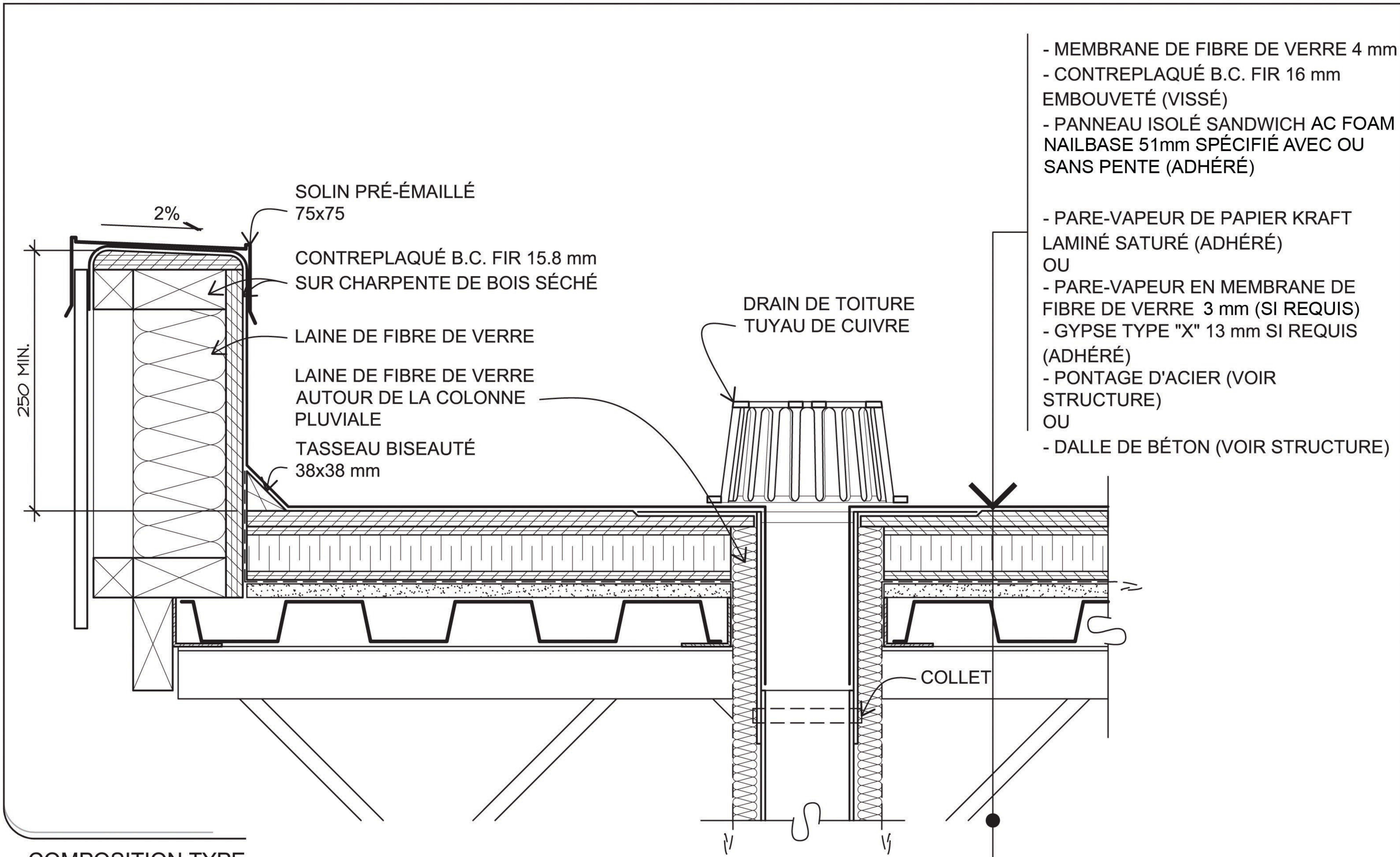
COMPOSITION TYPE TOITURE PLATE - PARAPET
